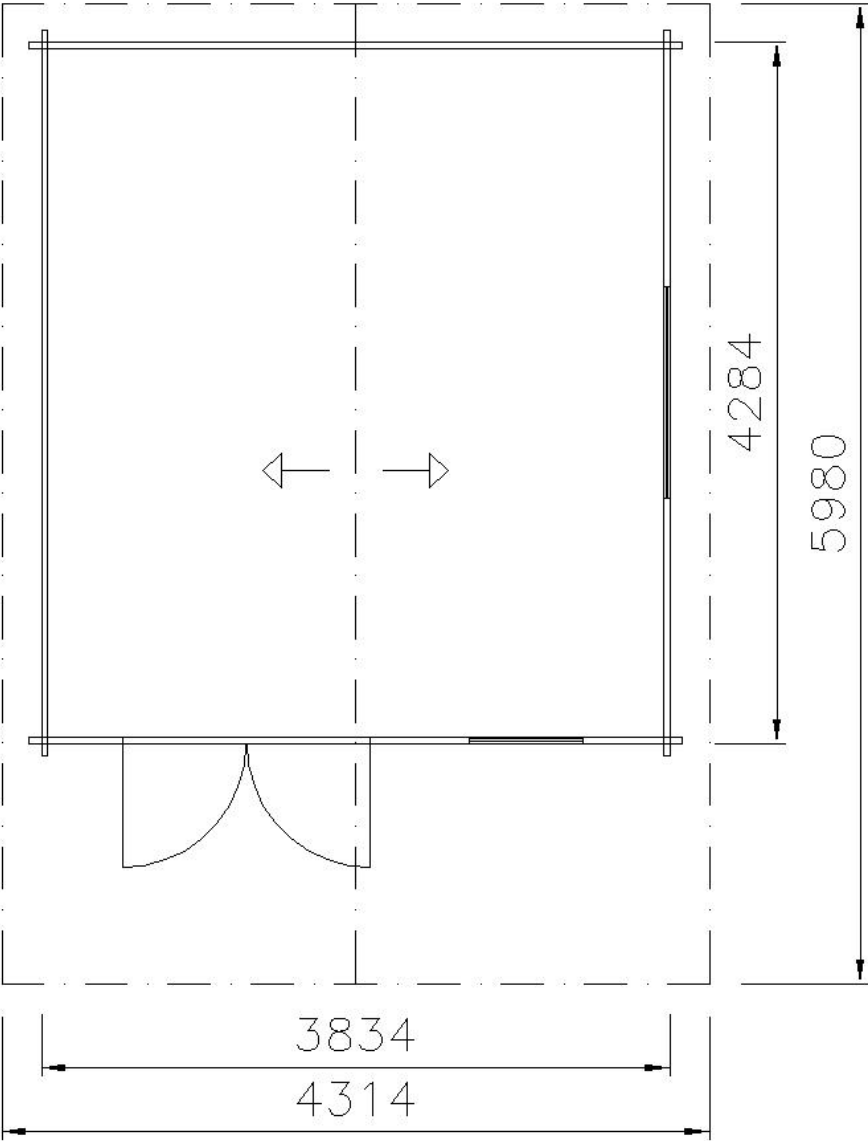
PÔDORYS
